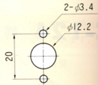
パネル穴明け寸法
