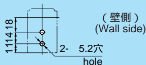
パネル穴明け寸法 Panel drilling dimensions
