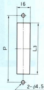
パネル穴明け寸法
