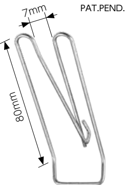
C-1624-1 ビニペット® 取付けタイプ
