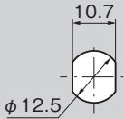
パネル穴明け寸法 Panel drilling dimensions
