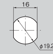
パネル穴明け寸法 Panel drilling dimensions
