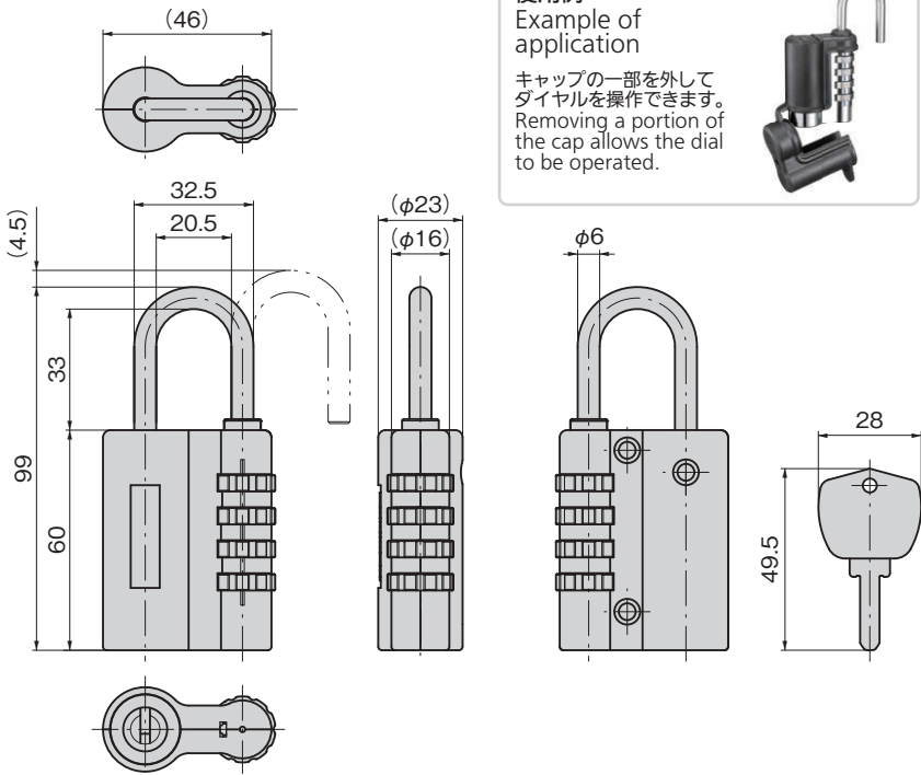
C-587-DL + C-587-DL-RC
