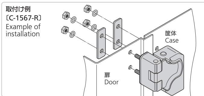
使用例 [C-1567-R] Example of application
