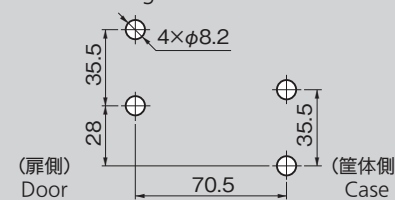
パネル穴明け寸法(C-1567-R) Panel drilling dimensions
