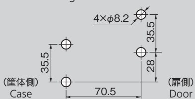
パネル穴明け寸法(C-1567-L) Panel drilling dimensions
