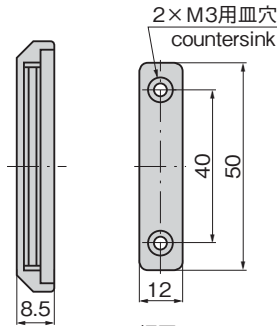
〔C-74用受板〕 Catch plate
