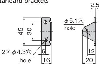
B-461-2~4用 標準ブラケット [B-461-A-2] Standard brackets
