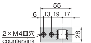
[ロッド棒ガイド] Rod guide
