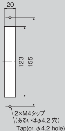
パネル穴明け寸法 Panel drilling dimensions
