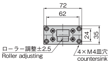
[ロッド棒ガイド] Rod guide
