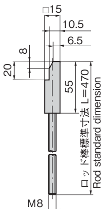
[ロッド棒] Rod
