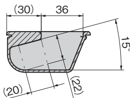
断面図 A-A Cross-section
