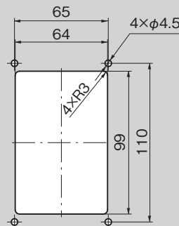
パネル穴明け寸法 Panel drilling dimensions
