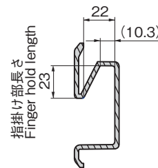
参考断面図 Reference cross-section
