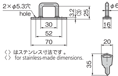
〔ストライカー〕 Striker
