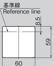
パネル穴明け寸法 Panel drilling dimensions
