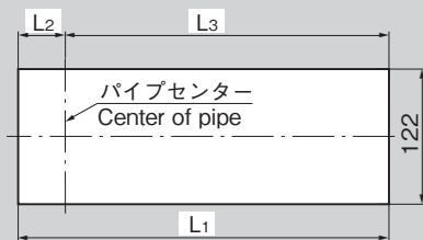
パネル穴明け寸法 Panel drilling dimensions
