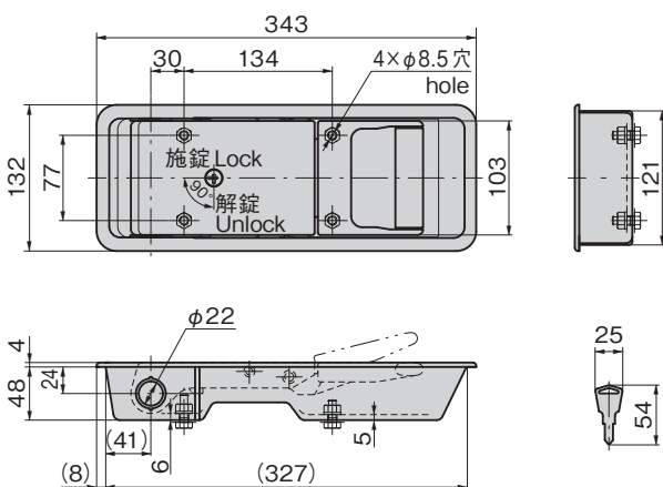
〔FA-877-1〕リア扉タイプ Rear door type
