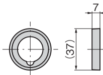
〔受座用キャップ〕 Base cap
