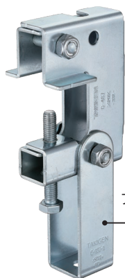
C-487-1 C-487-2より ブランコが23mm長い Swing is 23mm longer than C-487-2
