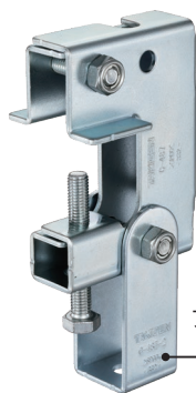
C-487-2 寸切りボルトを ブランコに取付けて使用 With full thread bolt mounted to swing
