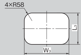
パネル穴明け寸法 Panel drilling dimensions
