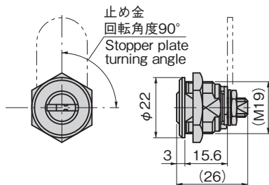
キーNo.TE1872 Key
