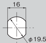
パネル穴明け寸法 Panel drilling dimensions
