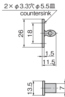
〔受け Base plate〕
