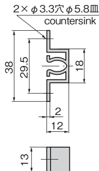
〔本体 Main body〕
