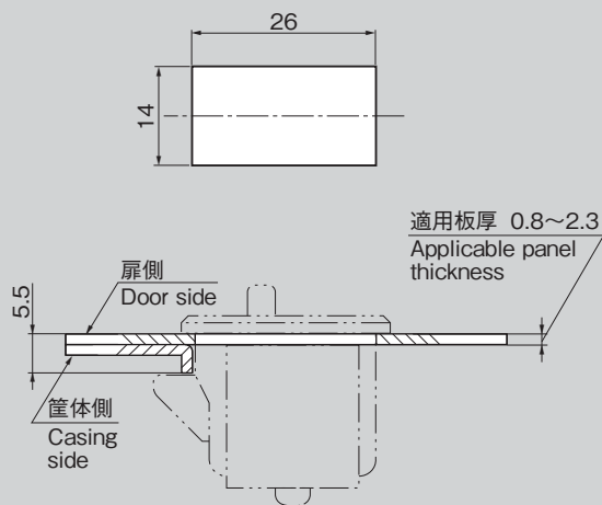
パネル穴明け寸法 Panel drilling dimensions
