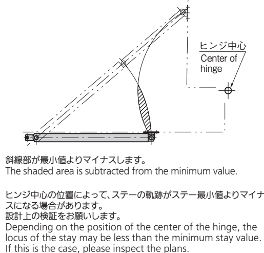
参考使用例 Example of application
