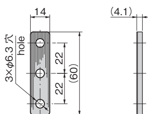
〔調整板〕 〔Adjustment plate〕
