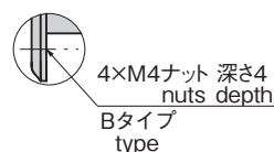
パネル穴明け寸法 Panel drilling dimensions
