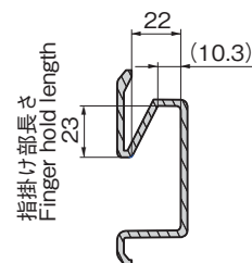
参考断面図 Reference cross-section
