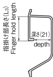
参考断面図 Reference cross section
