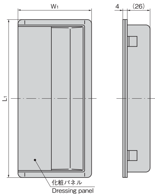
参考断面図 Reference cross section
