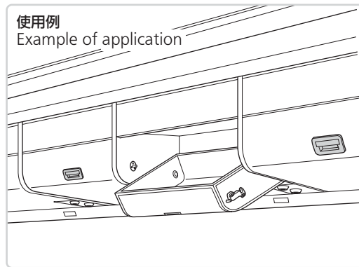
平面取付け用ブラケット Bracket for flush installation
