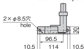
〔FA-1810-1B用フック・キーパー〕 Hook and keepers
