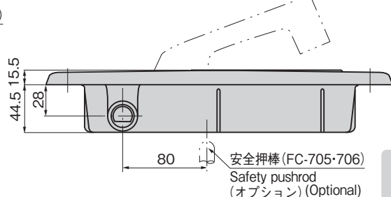
インジケーター (Lock: 生地色 Open: 赤色) Indicator (Lock: Plain color Open: Red color)
