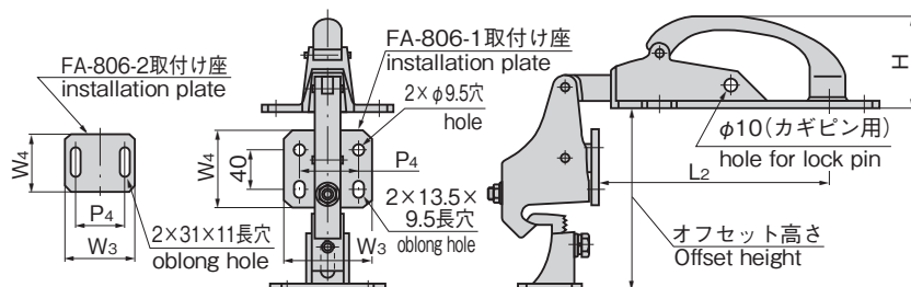
〔ハンドル本体〕 Handle main body
