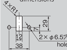
パネル穴明け寸法 Panel drilling dimensions
