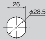
パネル穴明け寸法 Panel drilling dimensions
