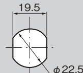
パネル穴明け寸法 Panel drilling dimensions
