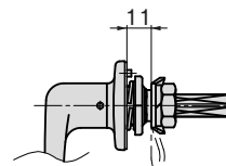
ナットAを使用しない場合 Without nut A
