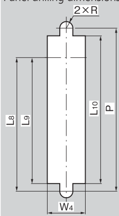
パネル穴明け寸法 Panel drilling dimensions
