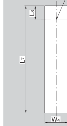
パネル穴明け寸法 Panel drilling dimensions
